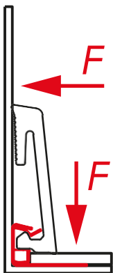
Opcja 1. (w trakcie kładzenia podłogi) Specjalny klips beznarzędziowy ze stali nierdzewnej
